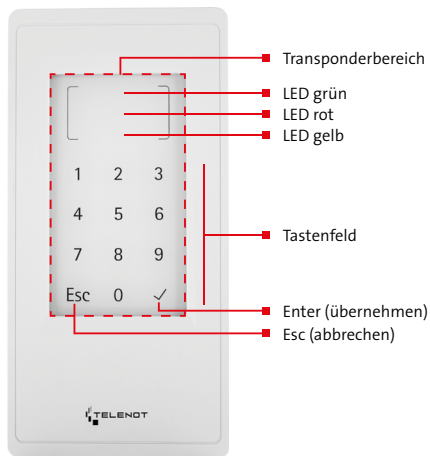
Aufbau Leser cryplock R/K-MD
